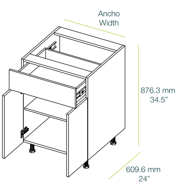
2 puertas - 1 cajón 2 doors - 1 drawer
