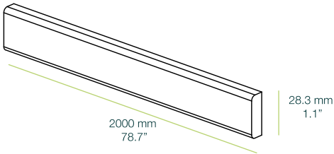
Moldura de ajuste - 9 mm / Scribe Molding - 0.3"
