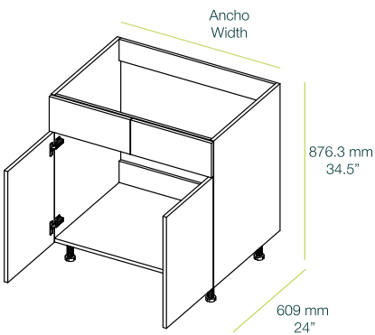
Mueble para fregadero - 2 puertas Sink base - 2 doors
