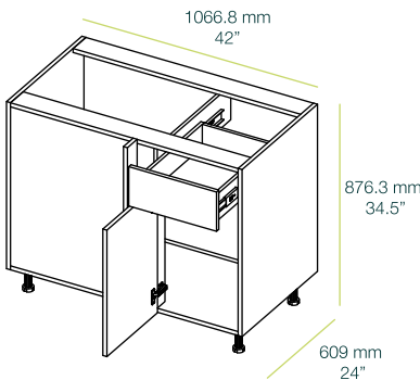
Esquinero ciego inferior 42\"/> Base blind corner 42\"/>
