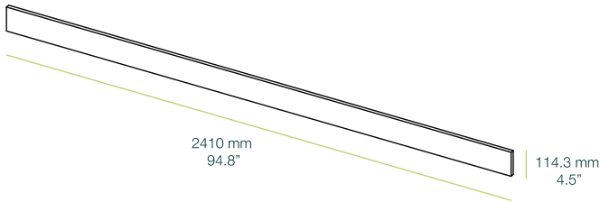
Zócalo - 18 mm / Toekick - 3/4"
