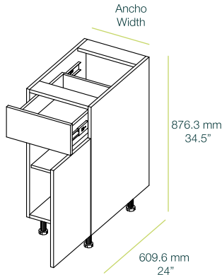
1 puerta - 1 cajón 1 door - 1 drawer
